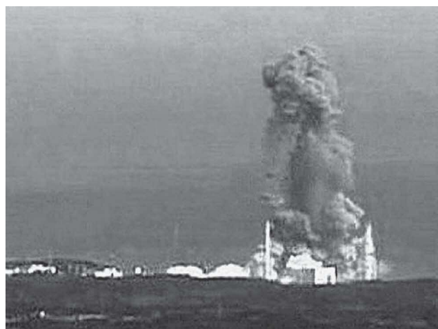
可燃性ガスも絡んでいた福島原発の爆発
